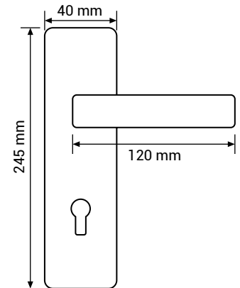
303245 mat siyah / matte black
