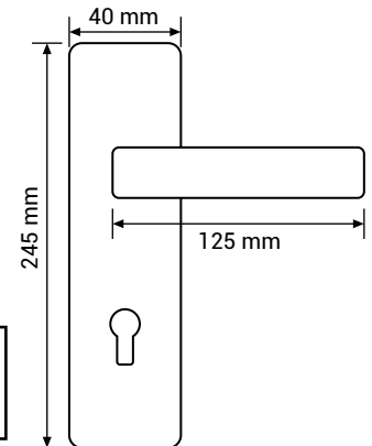
304245 mat siyah / matte black
